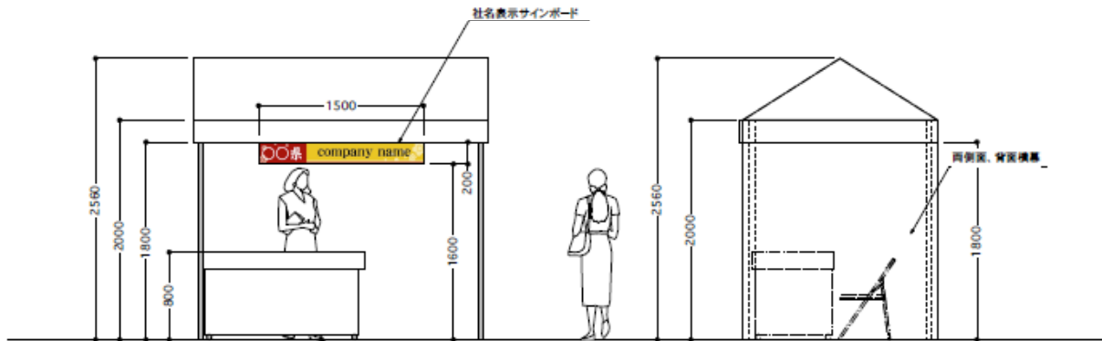
●立面図
