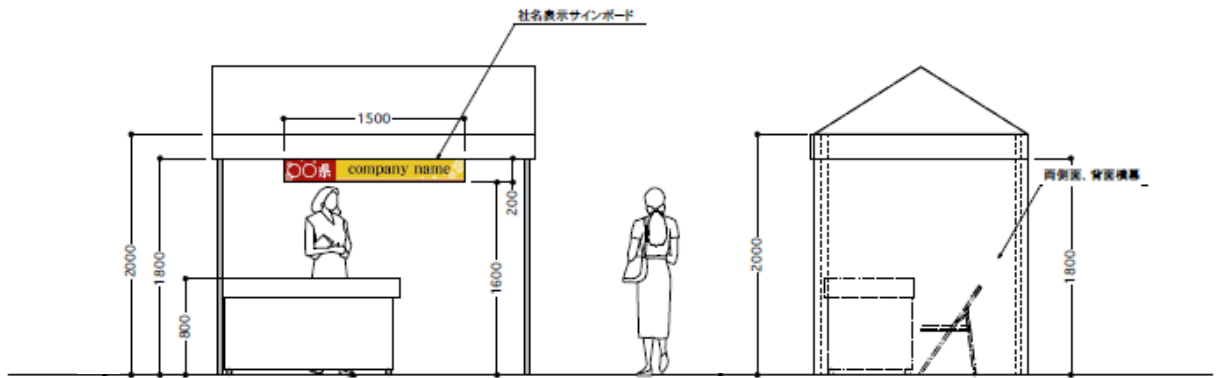
●立面図
